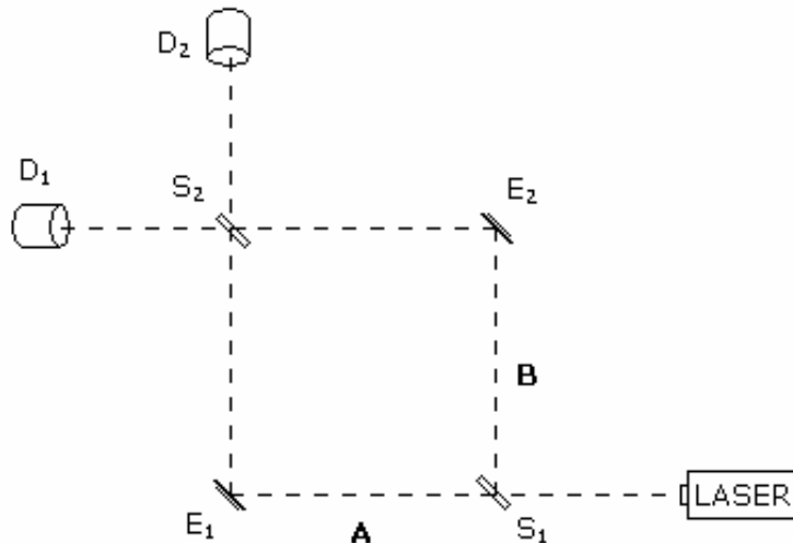
Figura 1.- Esquema do interferômetro de Mach-Zehnder.
