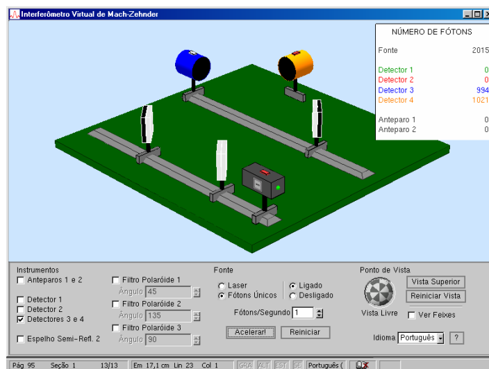
Figura 2.- Verificando a indivisibilidade dos fótons.
