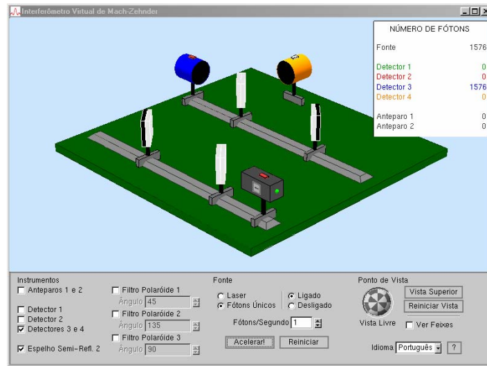
Figura 3. Interferência quântica com detectores
